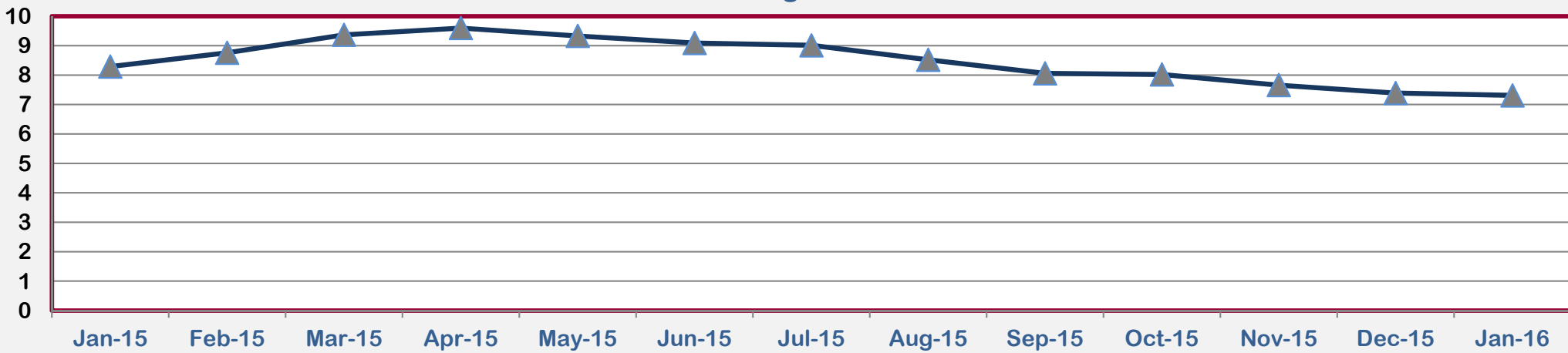
Region XIV
