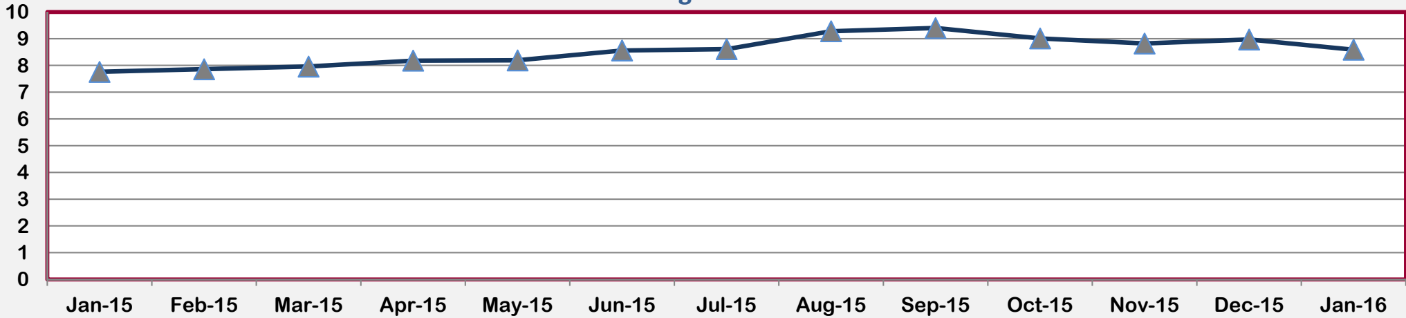
Region XIII
